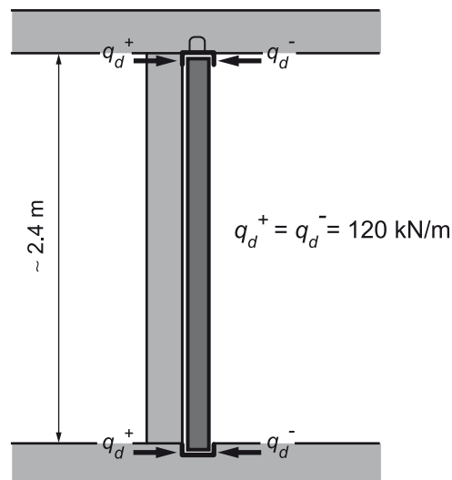
Abbildung 33 Horizontalkräfte bei Druckschiebewänden
