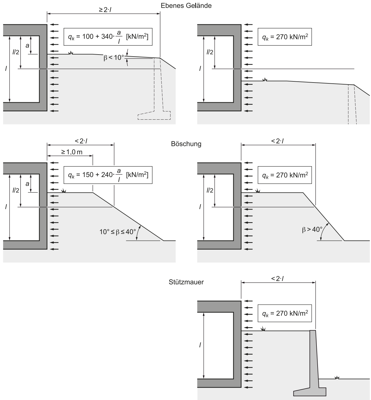
Abbildung 22 Einwirkung infolge Luft- und Erdstoss auf erdberührte Aussenwände bei mehrheitlich ebenem Gelände sowie bei Böschungen und Stützmauern
