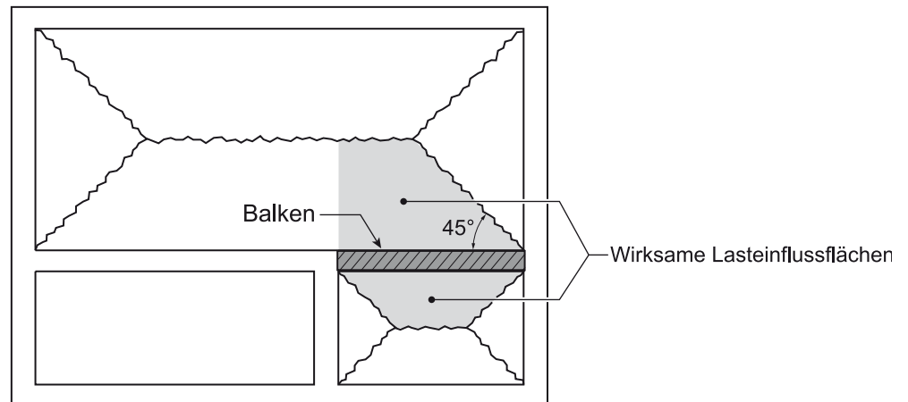
Abbildung 40 Balken als Plattenauflager bei einer einspringenden Ecke
