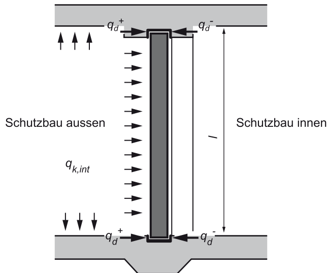
Abbildung 30 Auflagerkräfte von Panzerschiebewänden
