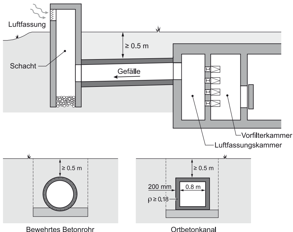
Abbildung 51 Luftfassungs- bzw. Abluftbauwerk
