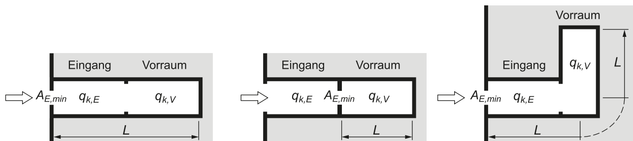
Abbildung 27 Konfigurationen von geschützten Eingangsbauwerken mit Korridoren
