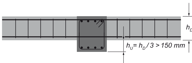
Abbildung 39 Plattenauflager mit Unterzug
