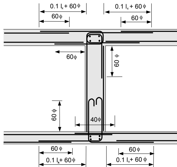
Abbildung 45 Bewehrung bei einer Wand zwischen zwei Schutzbauteilen (nur Biegebewehrung dargestellt)
