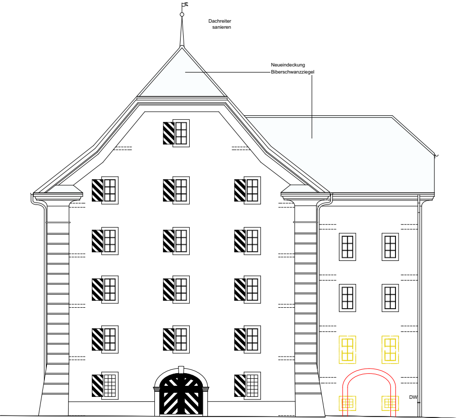
Ansicht Nord
