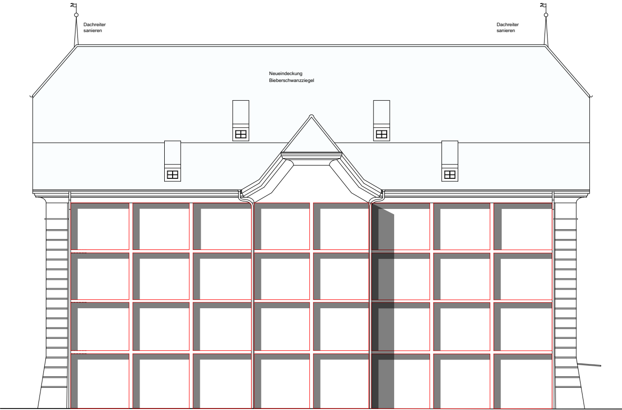
Ansicht West
