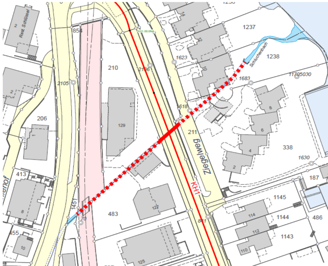
Legende: Situation mit Durchlasskanal (Auszug aus dem GIS; bearbeitet durch das Amt für Mobilität)
