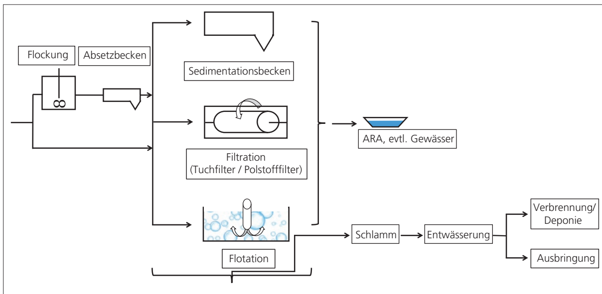
Abbildung 7: Übersicht über mögliche Verfahren zur Behandlung von erdreichen Abwässern
