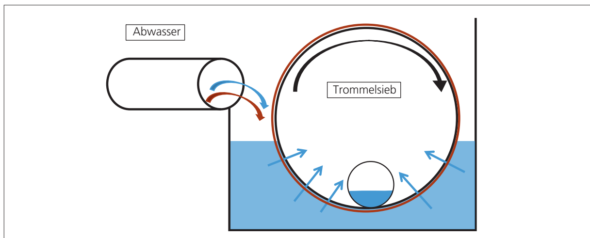
Abbildung 9: Trommelsieb zur Abscheidung von Feststoffen
