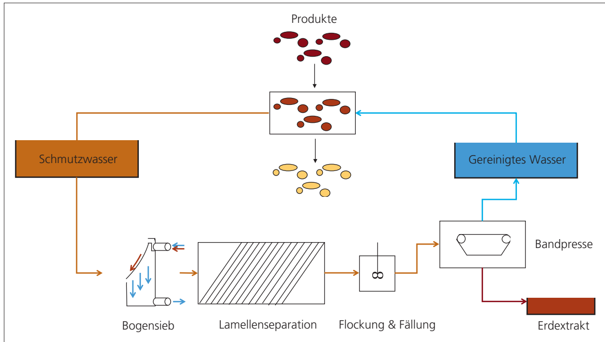
Abbildung 8: Schema einer kompakten Reinigung von erdhaltigen Abwässern
