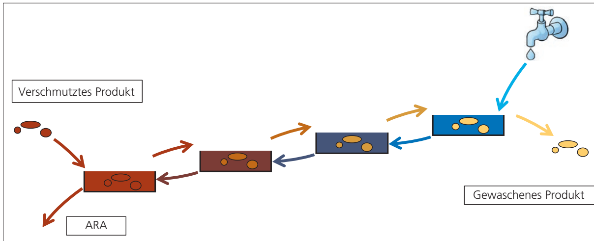
Abbildung 3: Kaskadenwaschsystem am Beispiel der Kartoffeln. Die Kartoffeln durchlaufen die einzelnen Becken von unten nach oben, das Wasser jedoch von oben nach unten.
