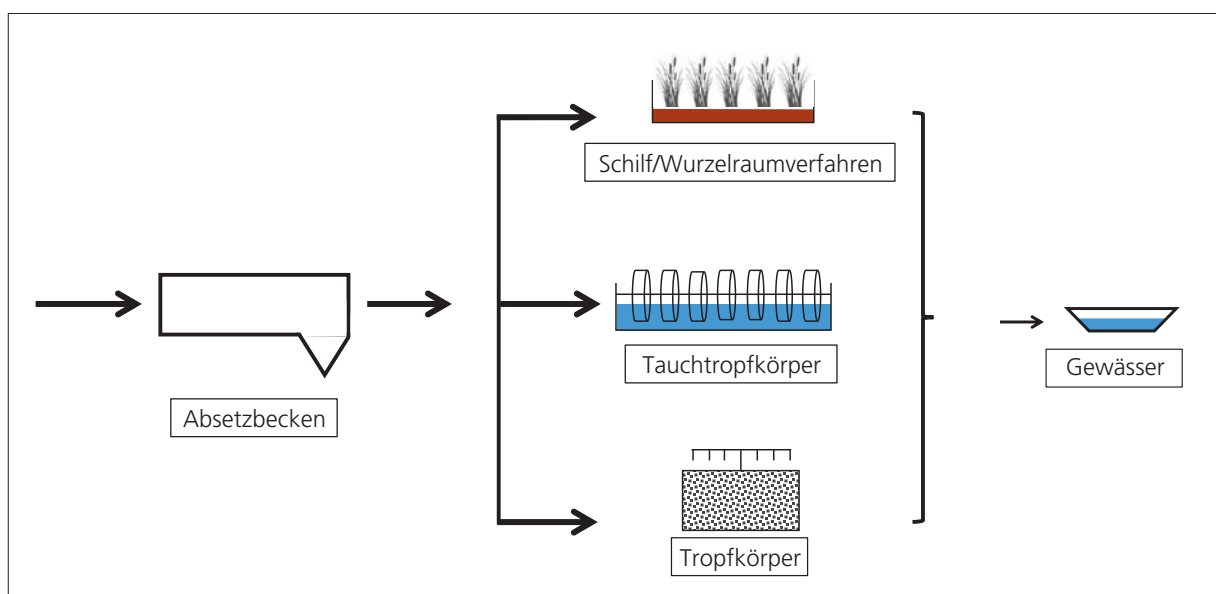
Abbildung 6: Übersicht über die Verfahren für leicht belastete Abwässer
