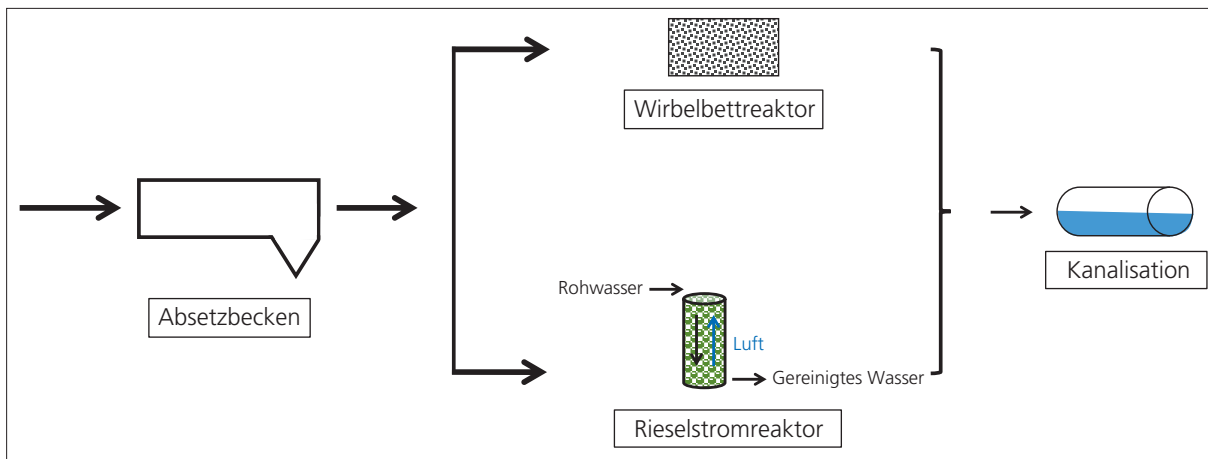
Abbildung 5: Grafik: tbfpartner Übersicht über die Verfahren bei mittel belasteten Abwässern, die nach der Vorreinigung in die Kanalisation eingeleitet werden
